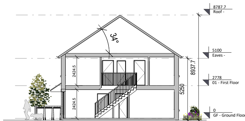
5 Section A-A 1 : 200
